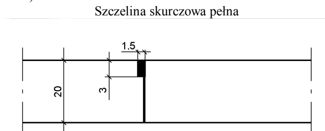
Rys. 1.1. Przykłady konstrukcji szczelin w podbudowie z betonu cementowego (wymiar w cm)
