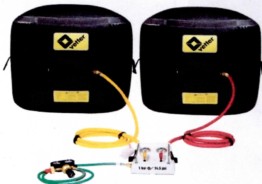
KW PSP w Łodzi - zestaw poduszek niskociśnieniowych Vetter 1/9.
