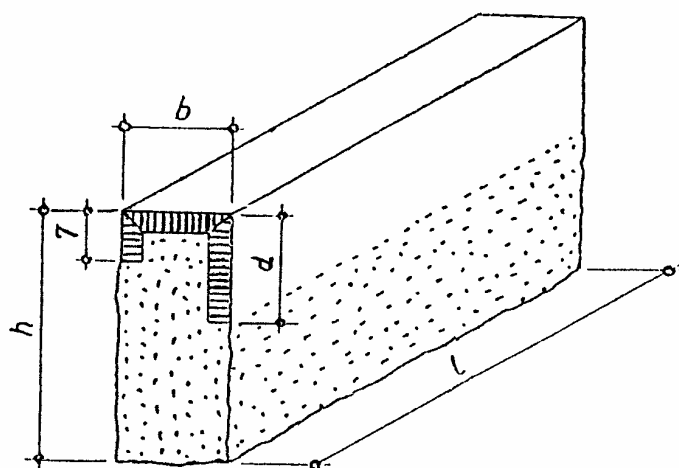
Rys. 1. Krawężnik uliczny odmiany UP, rodzaju B (opornik)
