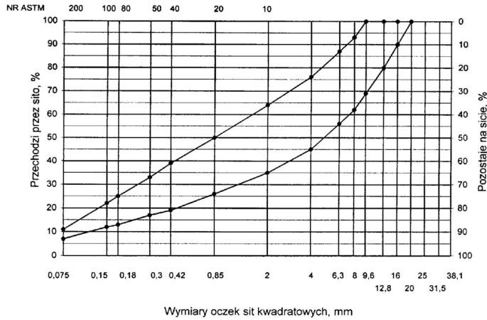
Rys 3 Krzywe graniczne uziarnienia mieszanki mineralnej BA od 0 do 20 mm do warstwy ścieralnej nawierzchni drogi o obciążeniu ruchem od KR3 do KR6
